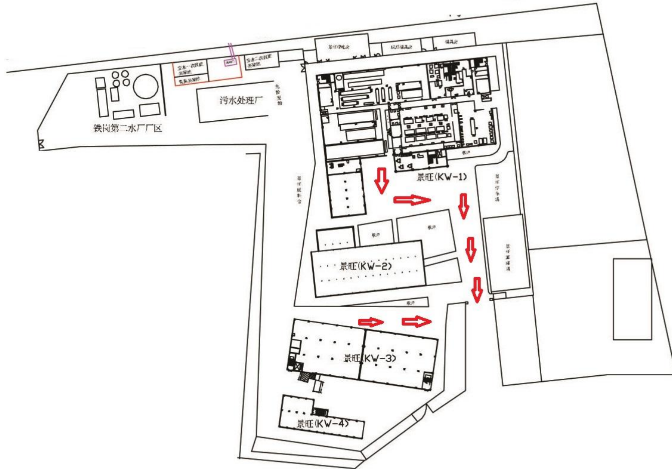
附图 5：厂区平面布置图及紧急疏散线路图
